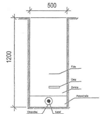
ŘEZ POD KOMUNIKACÍ
