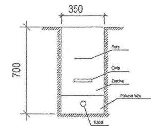
ŘEZ V TERÉNU
